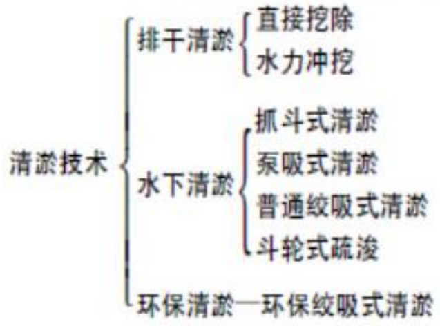
图 1-3 城市中小河渠清淤技术
