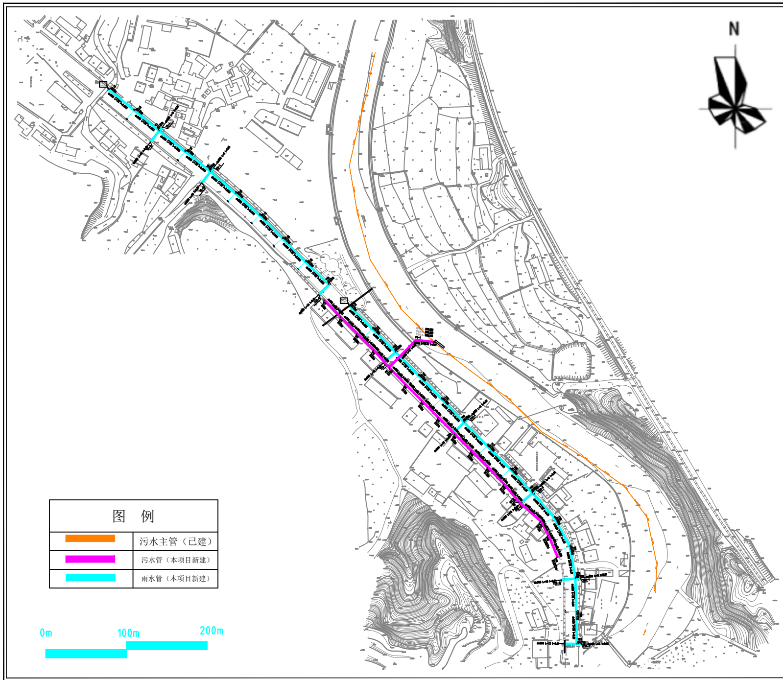
附图4 欧家河雨污管网治理方案总平面图
