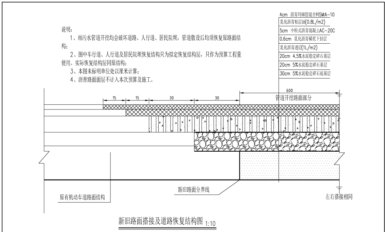
图 1-2 雨水管线道路面恢复示意图
